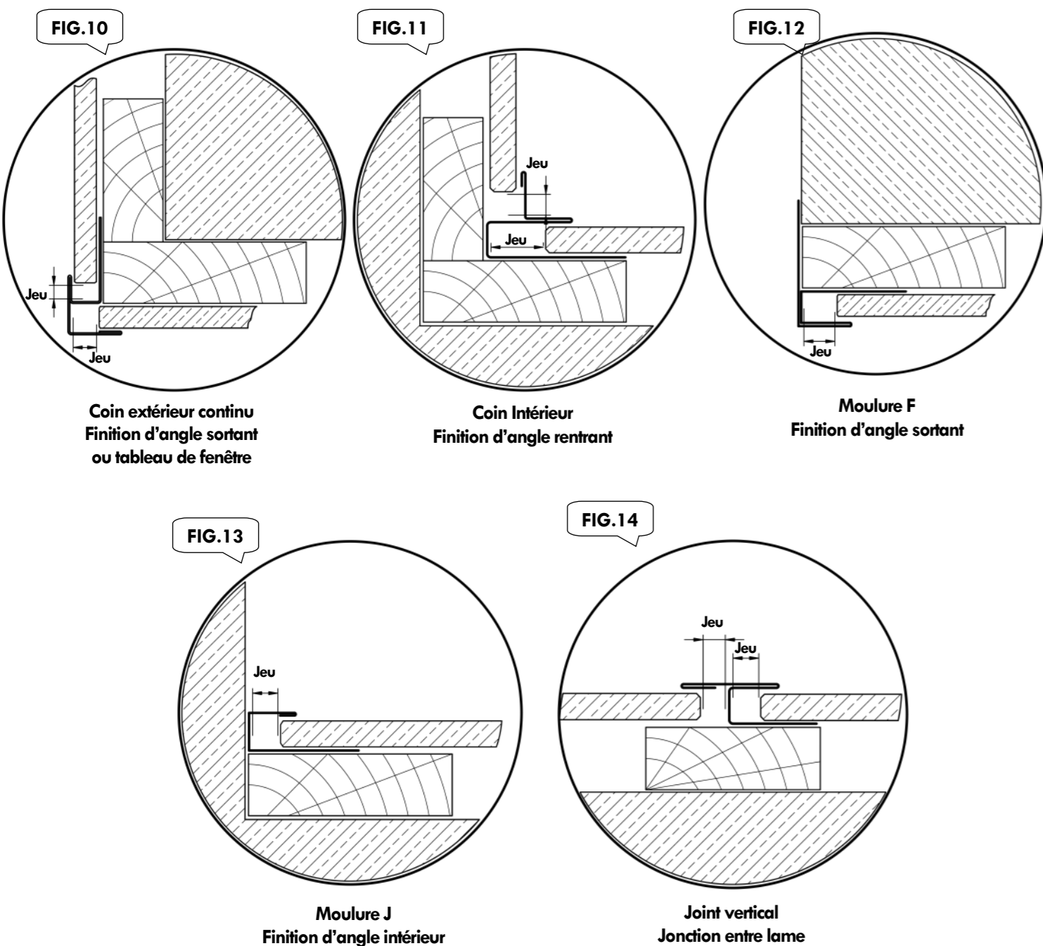
Fig.10 à 14 : Dilatation - Accessoires
