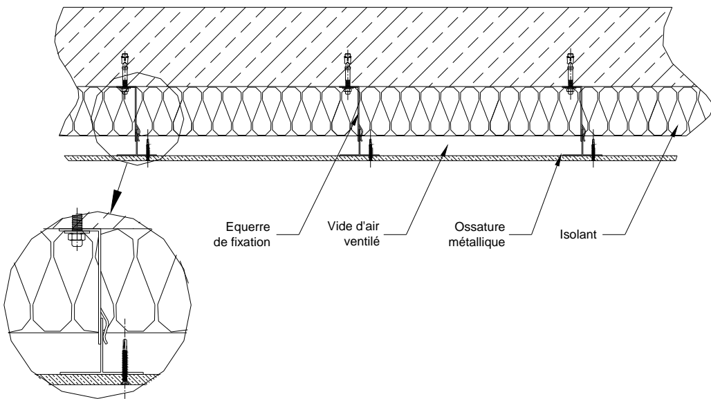
Figure 21 – Pose verticale des panneaux sur ossature métallique
