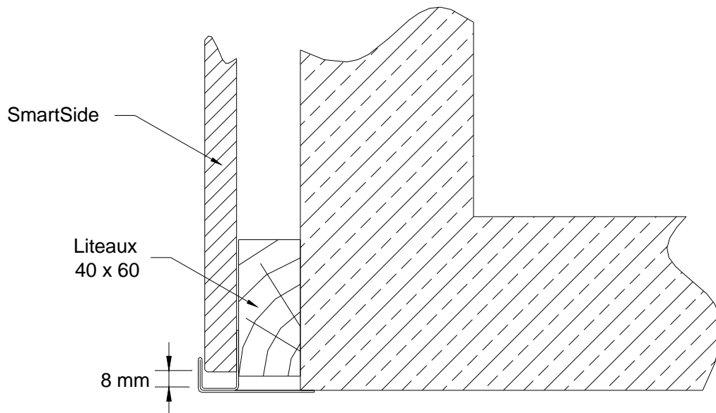
Figure 14 – Arrêt sur revêtement – Moulure F
