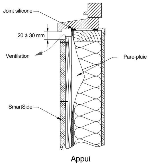
Figure 27 – Coupe sur menuiserie au nu extérieur de la MOB
