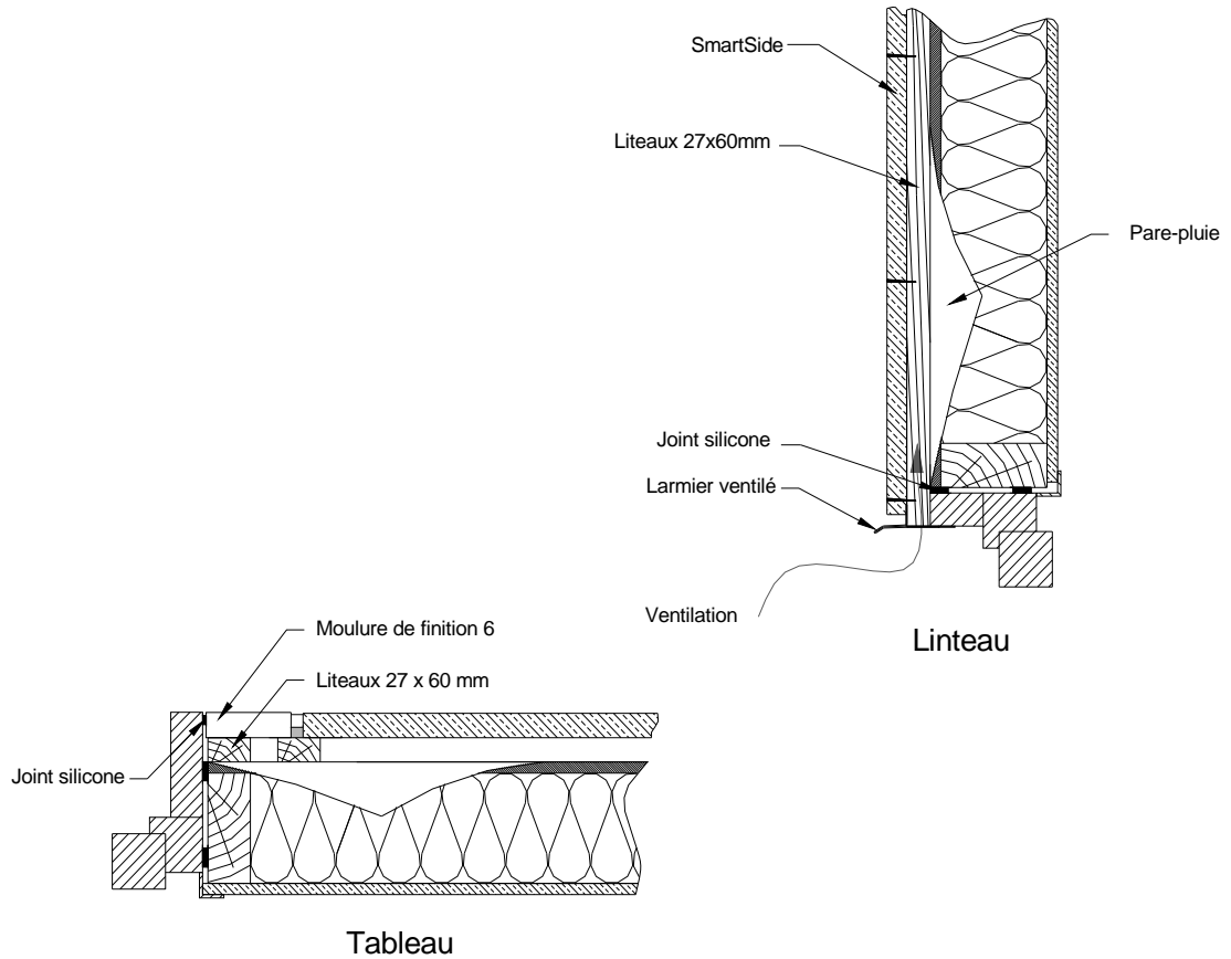
Figure 26 – Pose sur Maison Ossature Bois (coupe horizontale)
