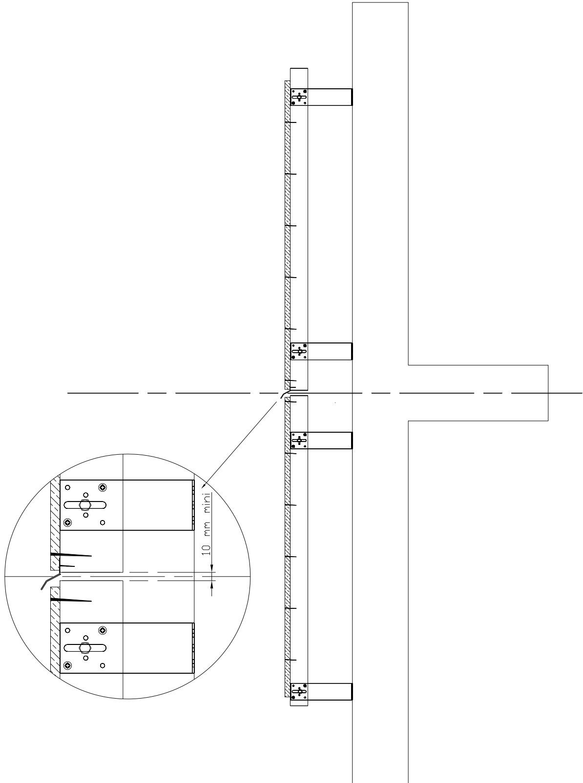
Figure A3 – Fractionnement au droit des planchers
