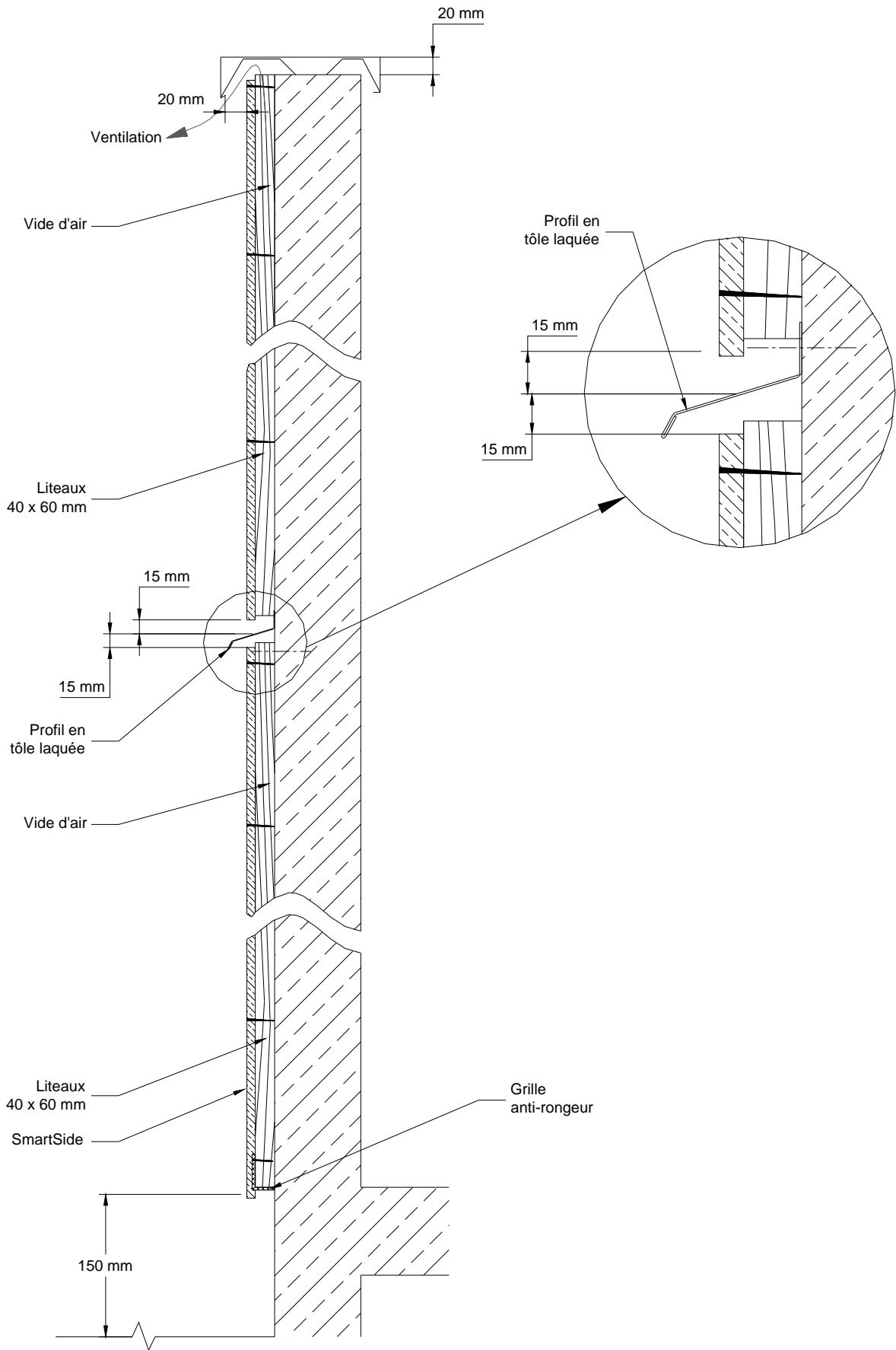
Figure 19 – Détails joint de fractionnement et acrotère
