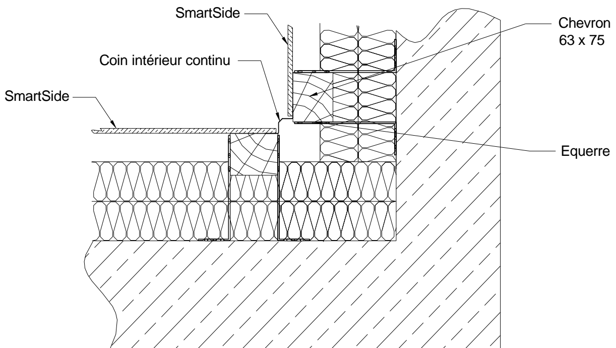
Figure 12 – Angle rentrant - Coupe sur isolant
