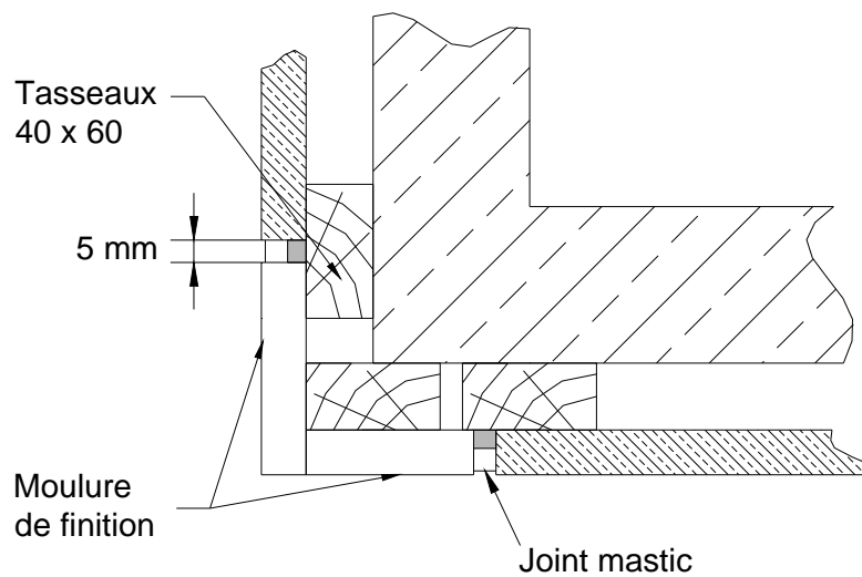
Figures 9 - Moulures de finition - Angle rentrant
