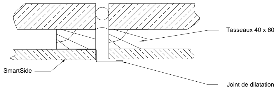
Figure 18 – Traitement du joint de dilatation longitudinal
