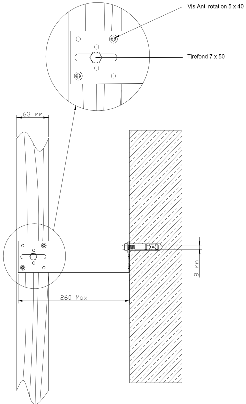
Figure A1 – Fixation de l'équerre sur le gros-œuvre – Fixation du chevron sur l'équerre
