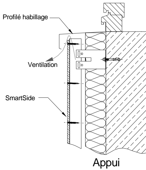
Figure 22 – Coupe sur menuiserie – Ossature métallique sur maçonnerie
