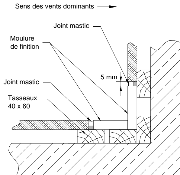
Figures 9 - Moulures de finition - Angle rentrant
