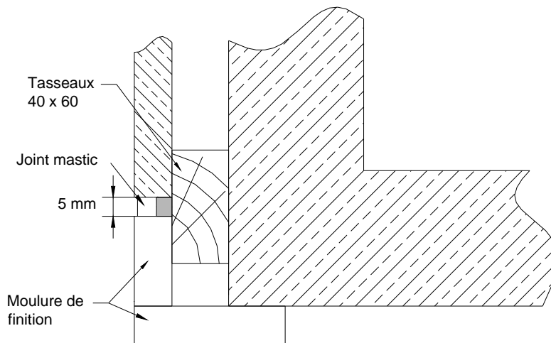
Figure 16 – Arrêt sur revêtement extérieur
