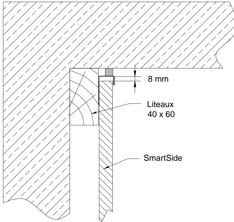
Figure 13 – Arrêt sur revêtement – Moulure J
