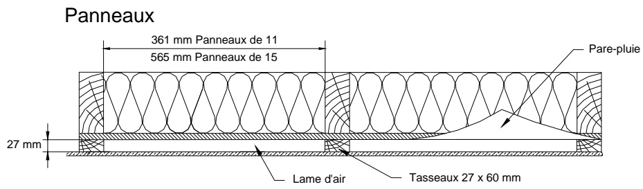
Coupe horizontale sur MOB - Panneaux
