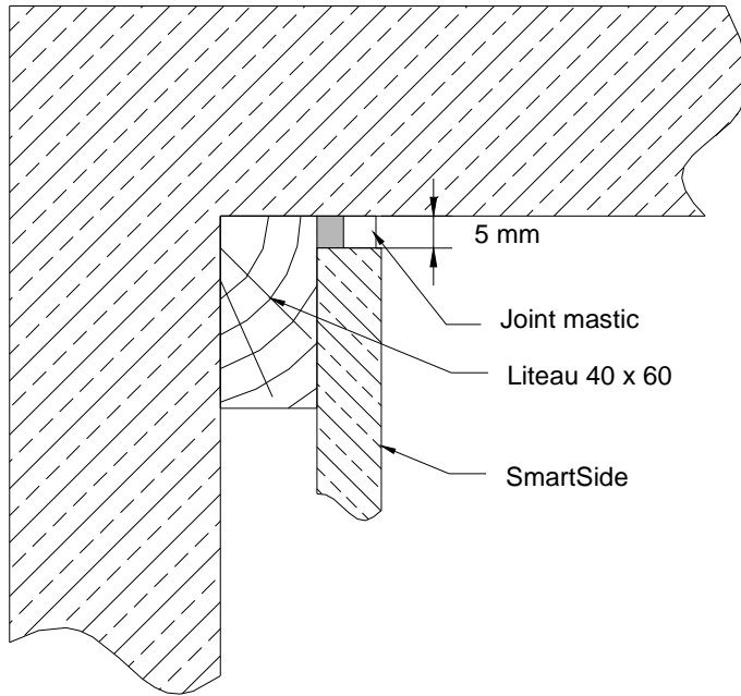
Figure 15 – Arrêt sur revêtement intérieur
