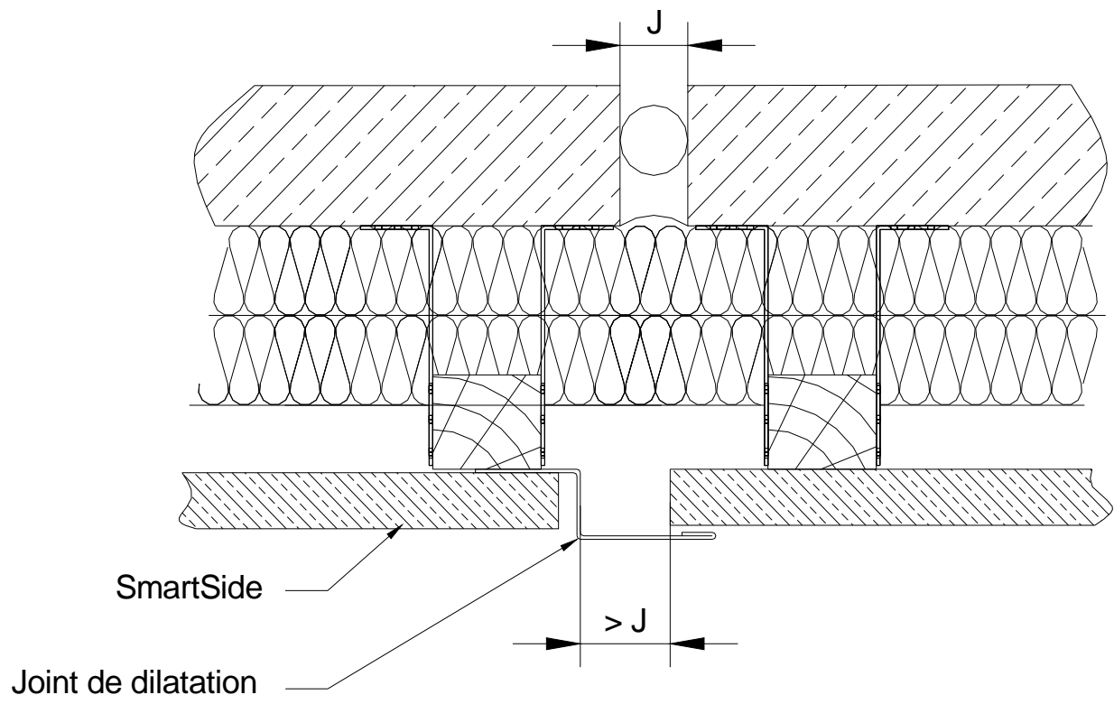
Figure A5 – Détail joint de dilatation 12 à 15 cm
