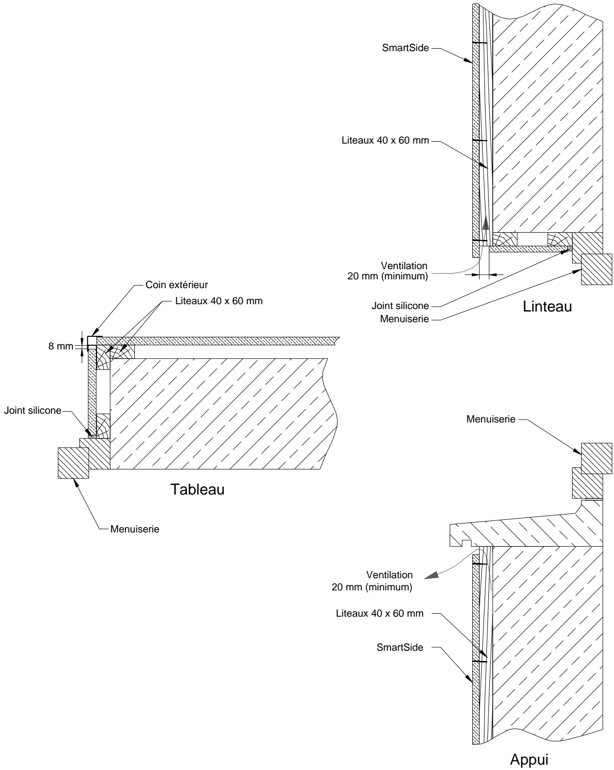
Figure 5 – Coupe sur menuiserie avec tableaux maçonnerie
