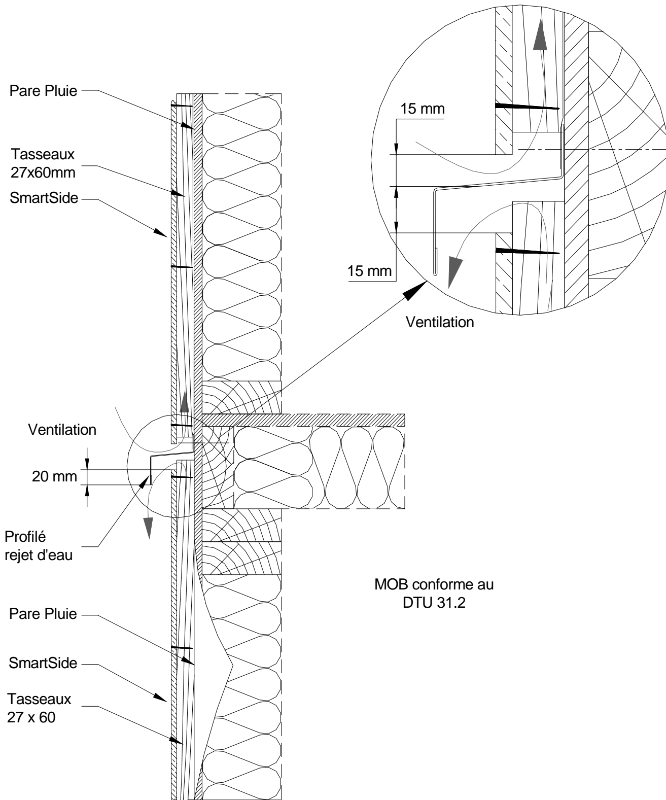
Figure A4 – Fractionnement plancher sur MOB
