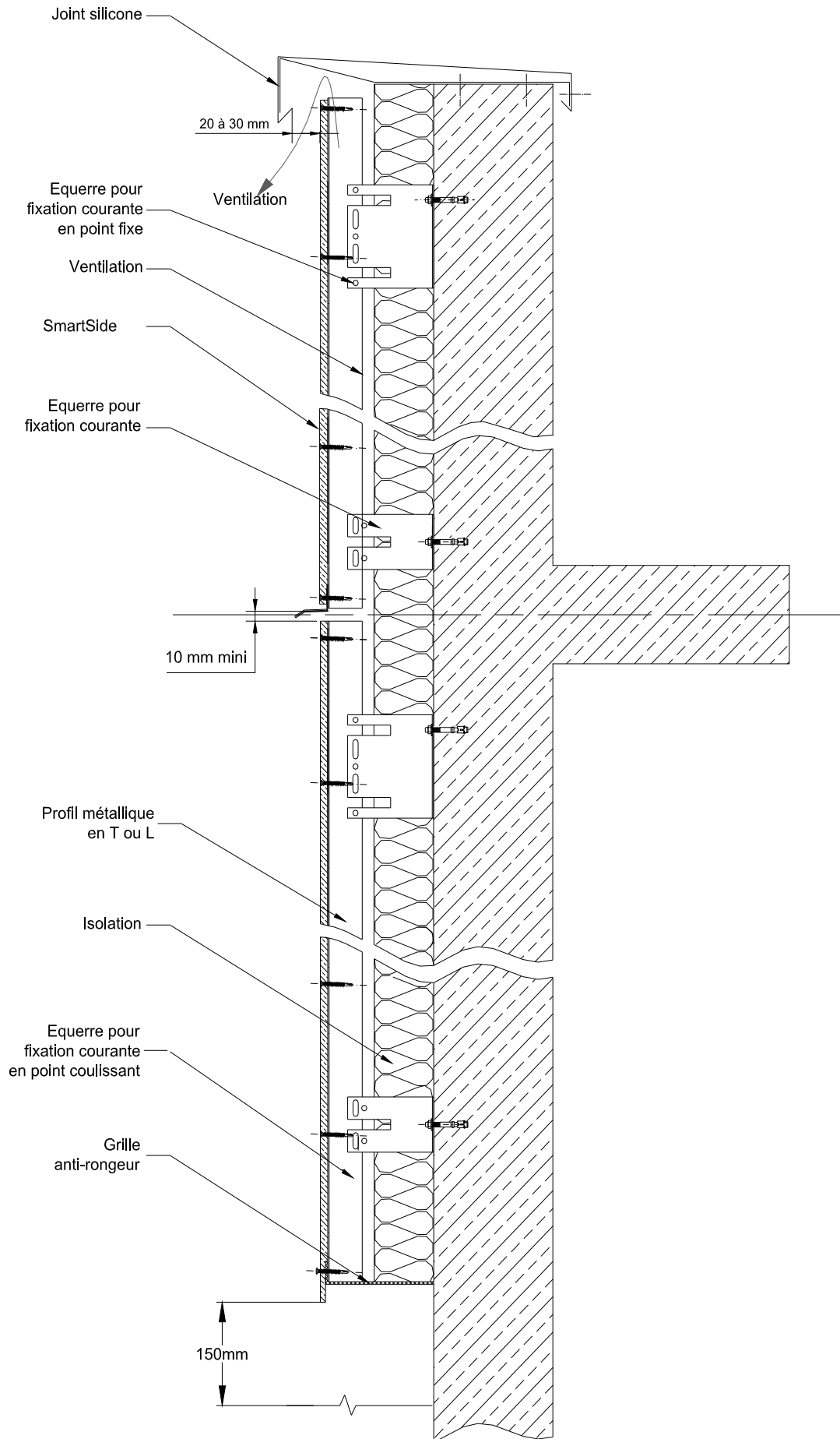
Figure 25 – Fractionnement de l'ossature
