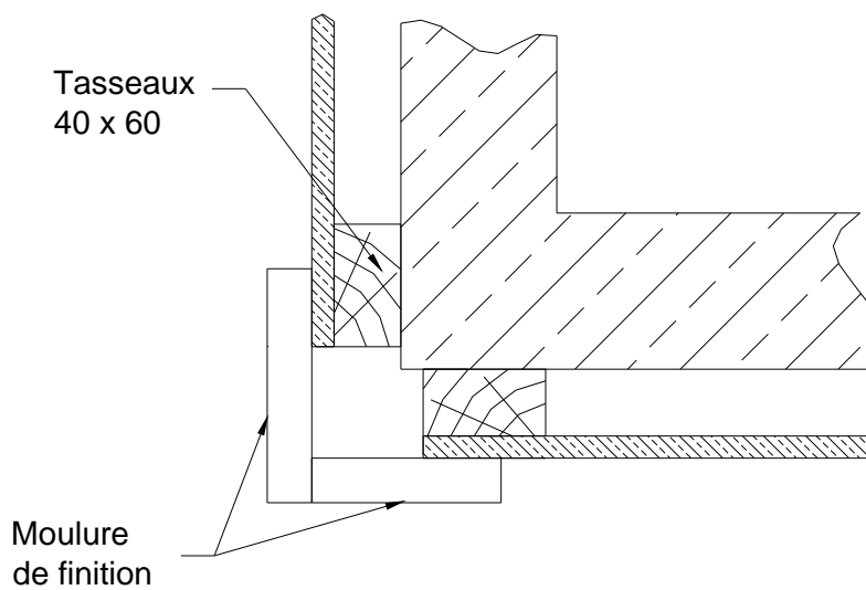
Figure 10 – Moulures de finition – Angle sortant
